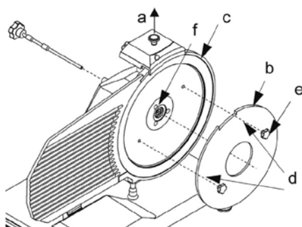
Fig. 7 – Zakładanie przyrządu z plexi (b) w celu zdjęcia noża
