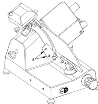
Εικ. 8 - Αποψη του εκτροπέα
