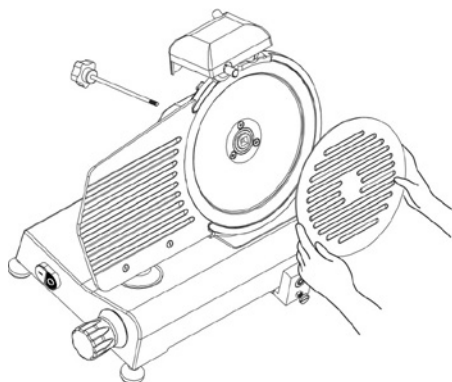
Rys. 6 – Zdejmowanie ostony noża
