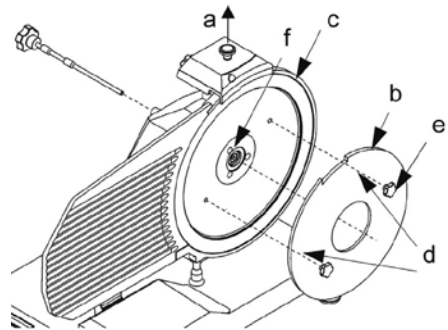
Εικ. 7 – Συναρμολογήστε το εργαλείο αφαίρεσης λεπίδας από Plexiglas (b)
