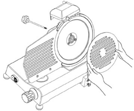
Εικ. 6 – Αφαίρεση προστατευτικού της λεπίδας
