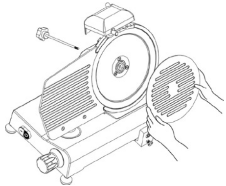
FIG. nr. 6 – Het losmaken van de beschermkap
