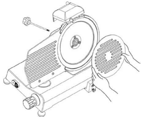
FIG. nr. 6 – Demontarea apărătoarei lamei
