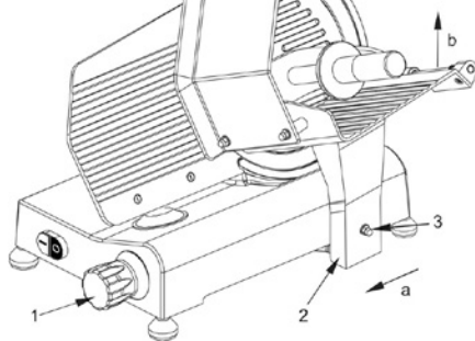
Разборка каретки.
