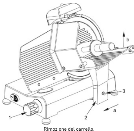
Rimozione del carrello.
