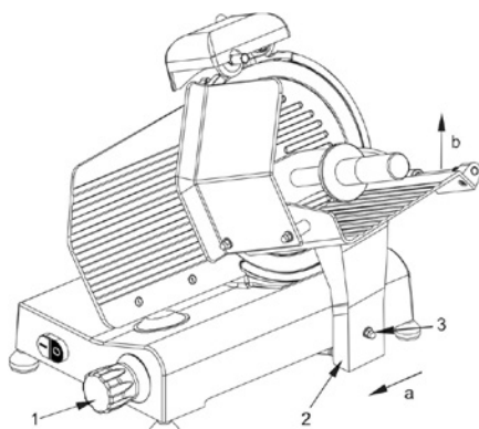
Zdemontowanie wózka.
